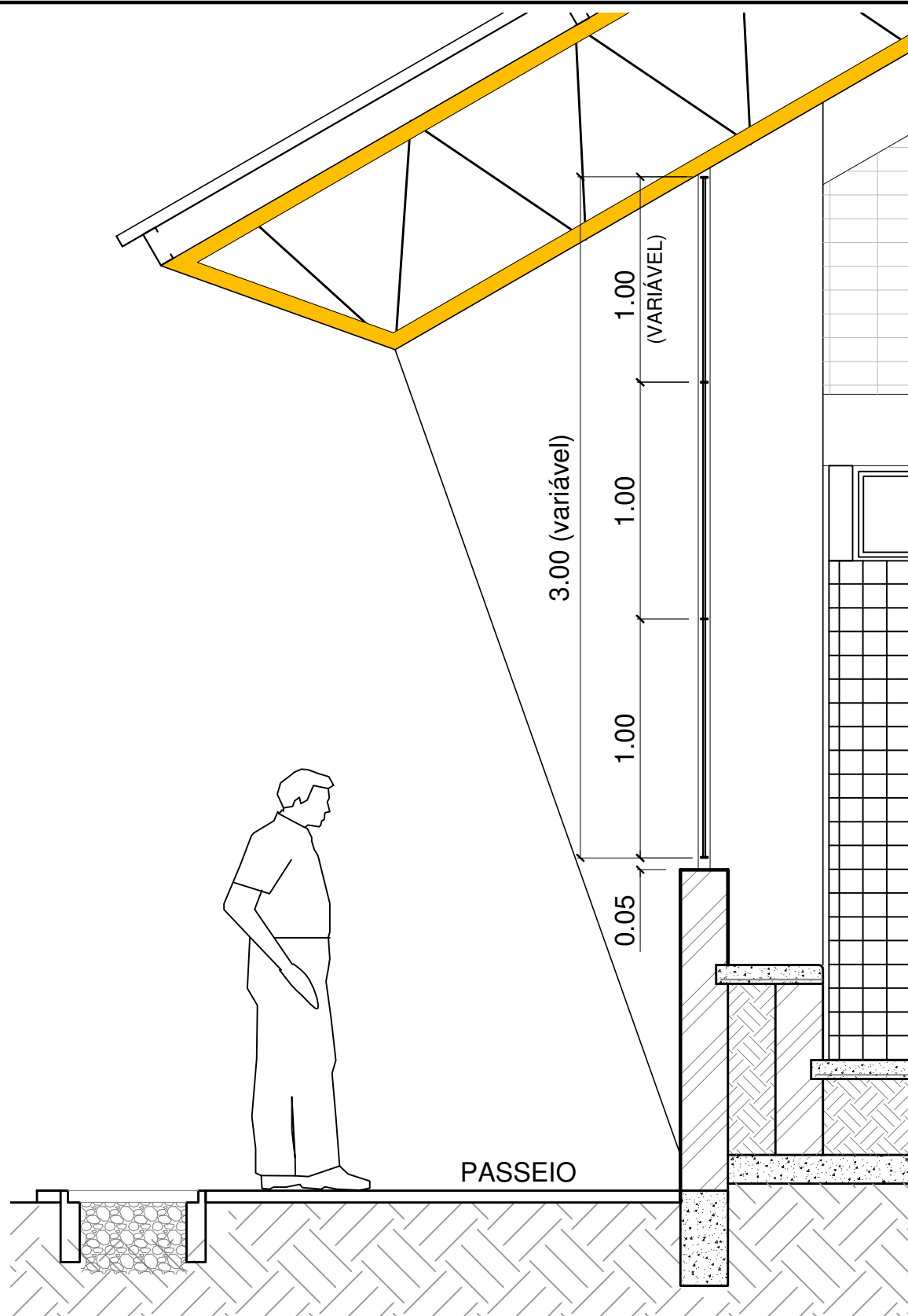
CORTE AA' Esc.: 1/25
