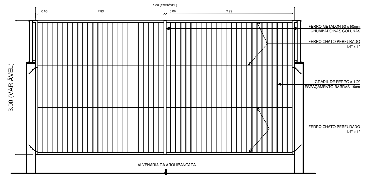
VISTA FRONTAL GRADIL PARA OS MODELOS: C - D - E - F - J - K - L - M Esc.: 1/50
